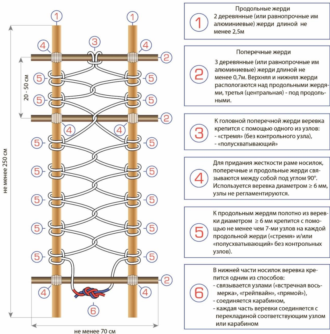
Рисунок 8.1 – Схема носилок
